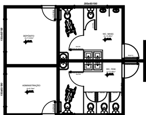
PLANTA BAIXA FUTURA
